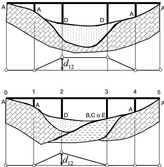
Figura 5.1. Esempi di insieme di spostamenti relativi da imporre ai supporti.
