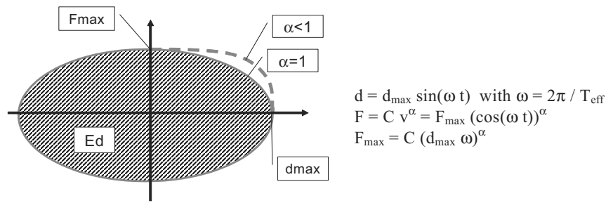
Figura 9.2 – Dispositivi a comportamento viscoso
